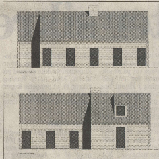
Sådan ser facadetegningerne til det kommende konfirmandhus ud.
